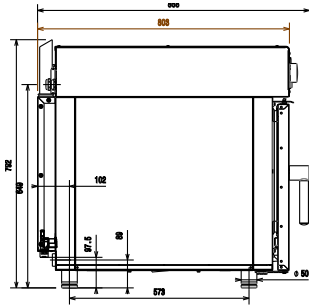
Oldalnézet
